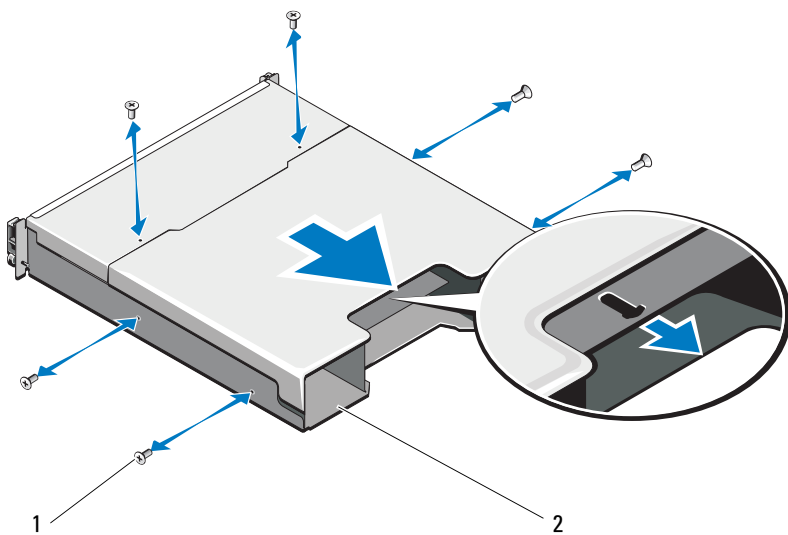
图 16-15. 卸下和安装 RAID 控制器模块 / 电源设备固定框架
